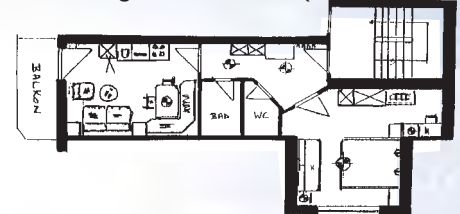
Wohnung für 2 - 3 Personen (45 m 2 )
